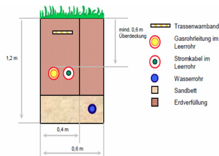
Bild 2: Stufengraben
